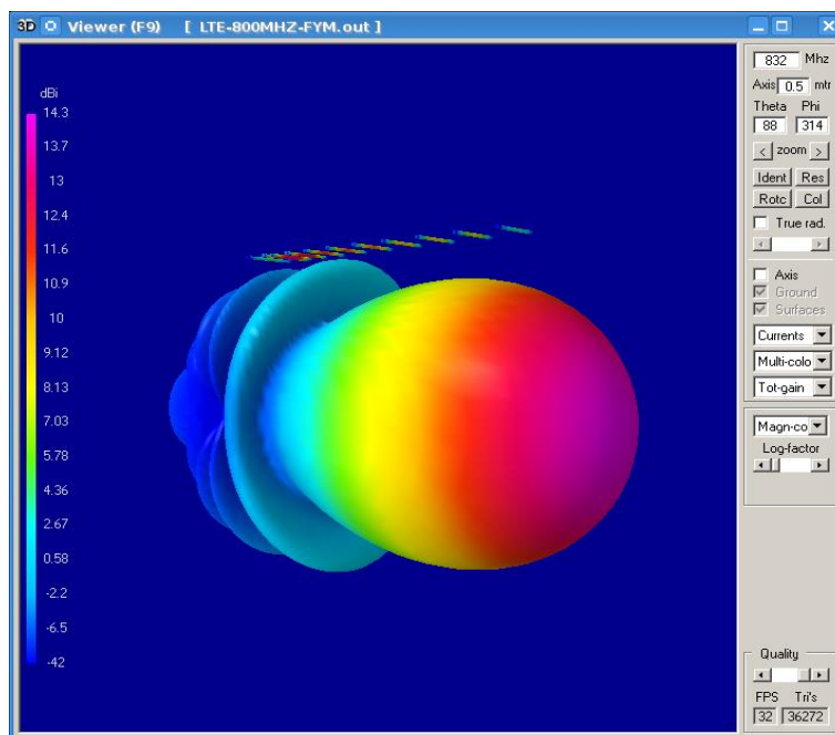
Figuur H.1: Berekend 832 MHz stralingspatroon van de Yagi in free space. Gain is ca. 13.6 +/- 0.7 dBi tussen 791 – 862 MHz
